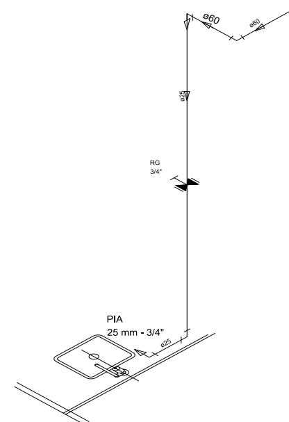
DETALHE H6 ESC.: 1:50
