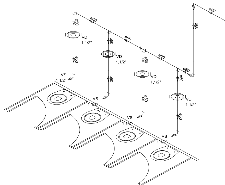
DETALHE H4 ESC.: 1:50
